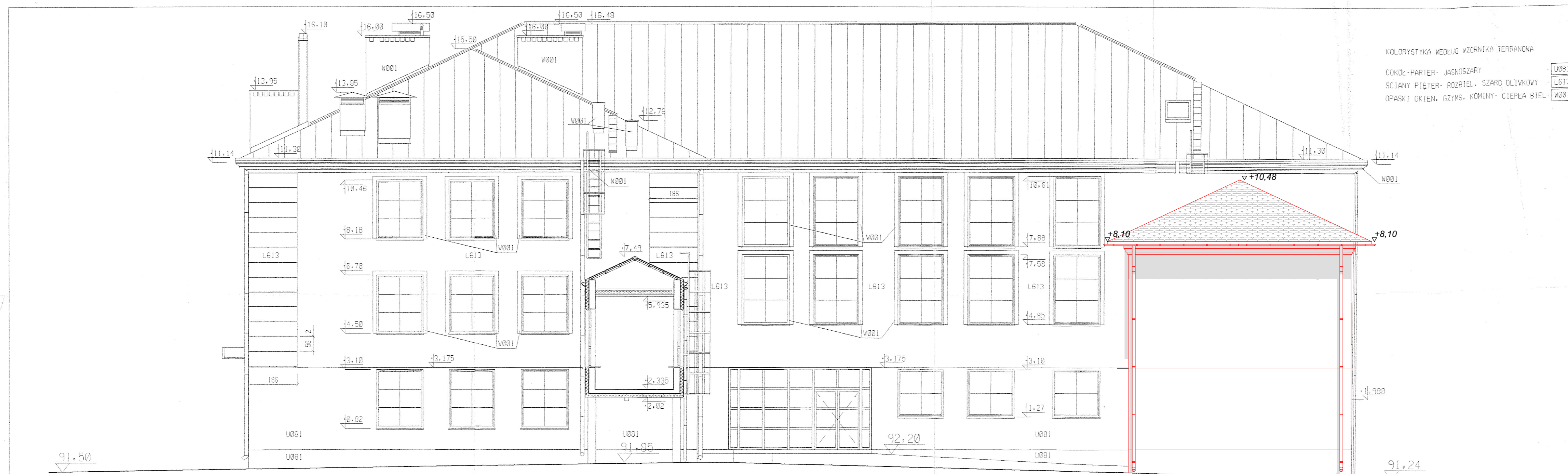
ELEWACJA PÓŁNOCNO ZACHODNIA
